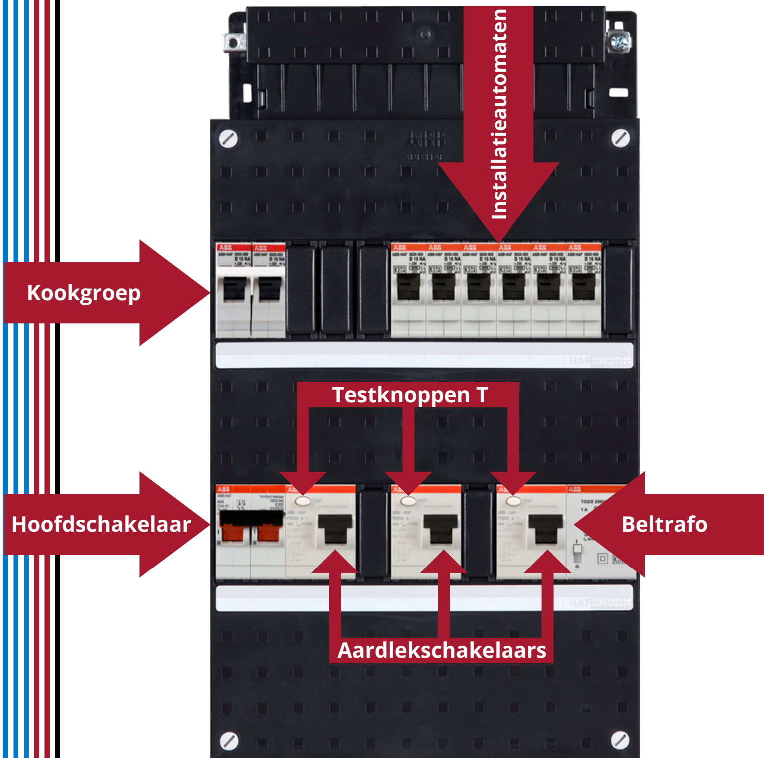
Afb. 1. Meterkast
